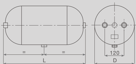
Luftbehållare med fyra hål M22x1,5
